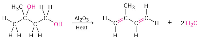
3-Methyl-1,3-butanediol
