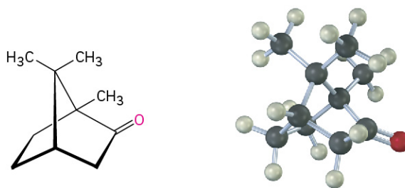
Camphor
