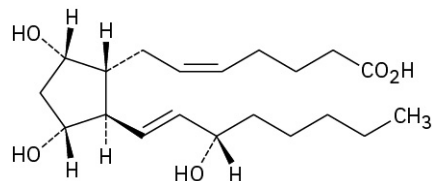
Prostaglandin F_{2\alpha}
