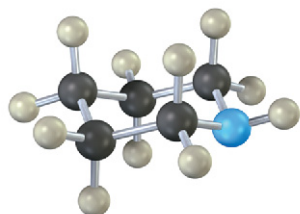
Piperidine
