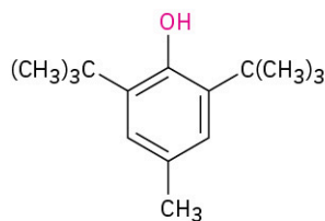
BHT
