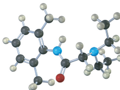
Lidocaine
