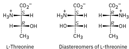
L-Threonine
