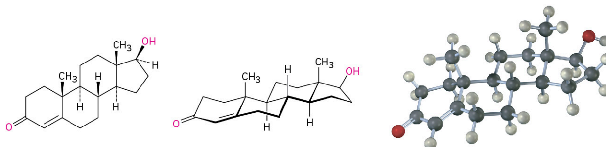
Testosterone (a steroid)
