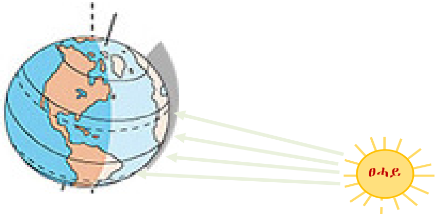
ስእሊ 2.9 ሓጋይ ኣብ ሰሜን ንፍቀ ክበ.
