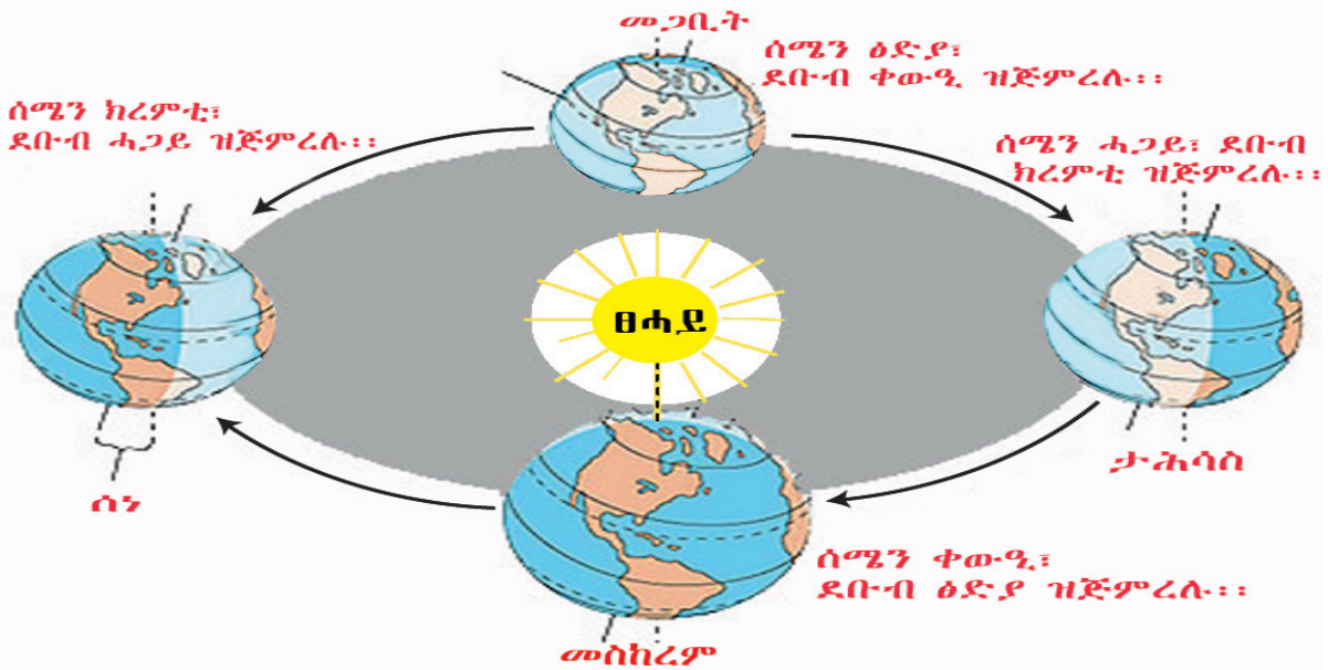
ስእሊ 2.10 ኣርባዕተ ወቐትታት ምድሪ
