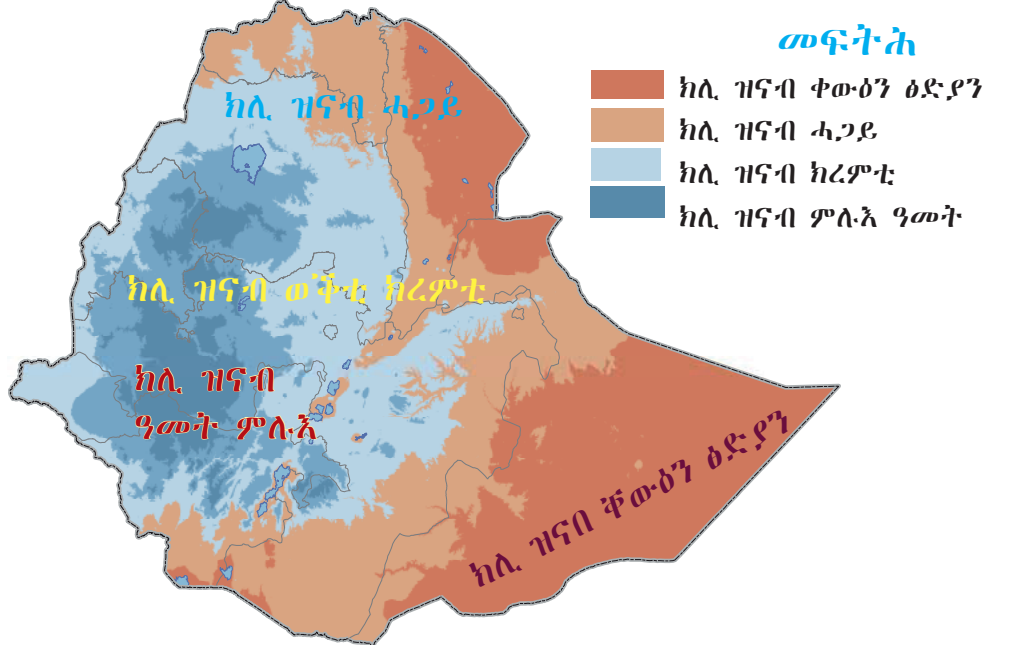
ካርታ 2.1 ክልታት ዝናብ ኢትዮጵያ፡፡
